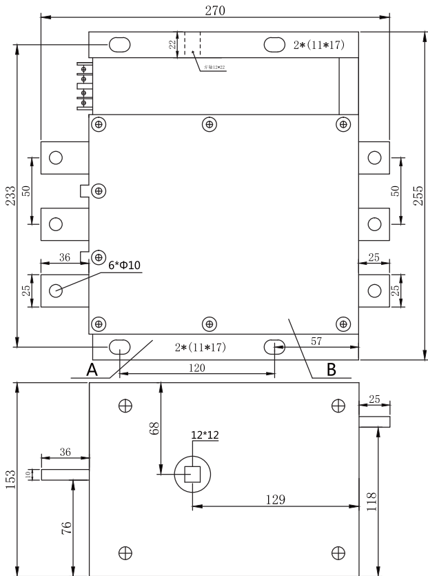
图6 BRGHK-500/1140隔离器（卧式操作）外形尺寸及安装尺寸（mm）
