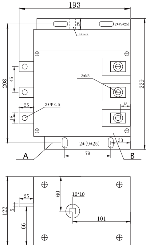
图1 BRGHK-200/1140隔离器（立式操作）外形尺寸及安装尺寸（mm）
