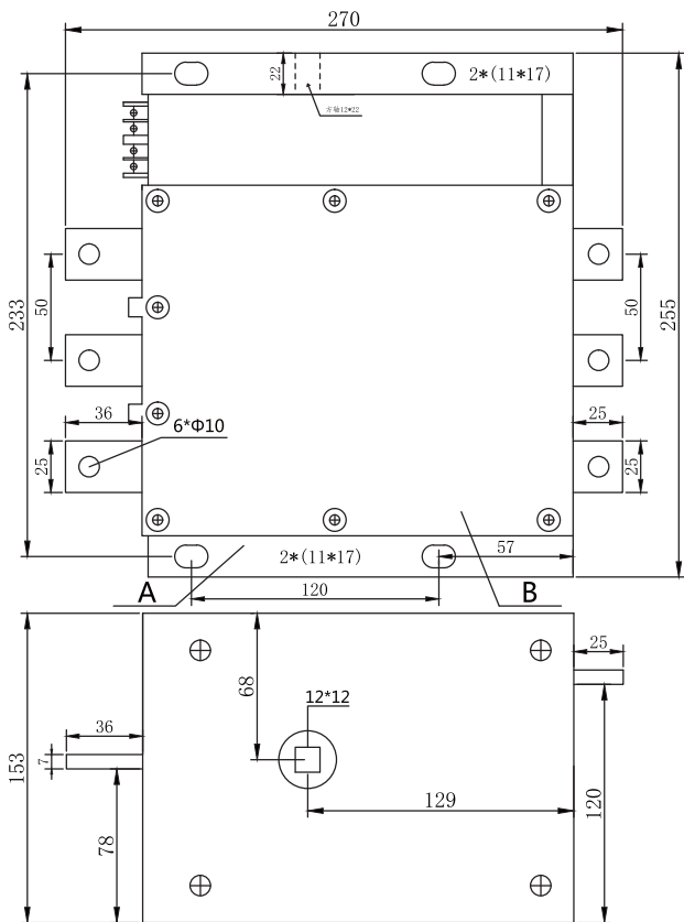
图4 BRGHK-315、400/1140隔离器（卧式操作）外形尺寸及安装尺寸（mm）
