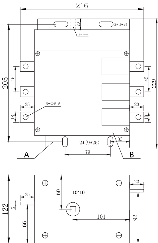
图2 BRGHK-200/1140隔离器（卧式操作）外形尺寸及安装尺寸（mm）
