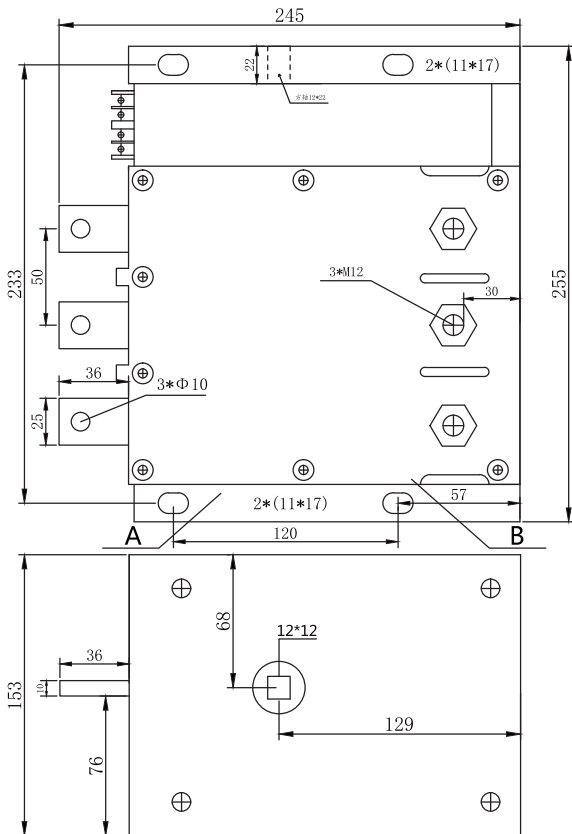
图5 BRGHK-500/1140隔离器（立式操作）外形尺寸及安装尺寸（mm）
