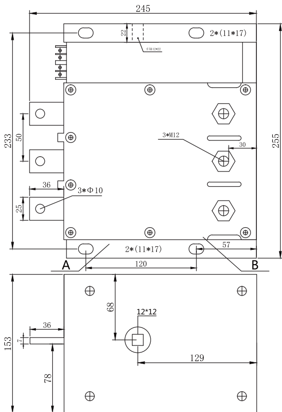
图3 BRGHK-315、400/1140隔离器（立式操作）外形尺寸及安装尺寸（mm）
